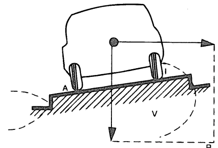
GRÁFICO 27: Peralte o sobreelevación.
