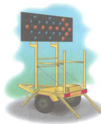
GRÁFICO 26: Señal luminosa transitoria.
