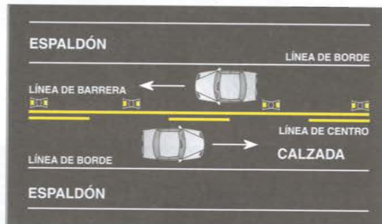
GRÁFICO 9: Línea de barrera.
