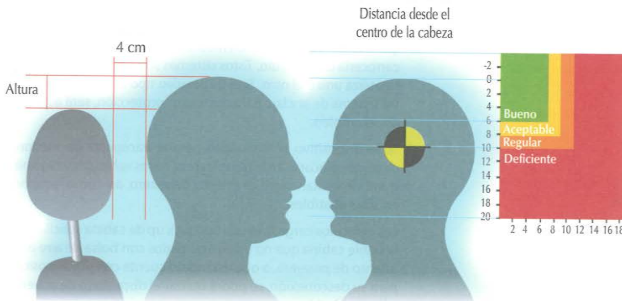
GRÁFICO 43: Apoya cabezas.
