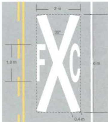
Cruce ferrocarril
