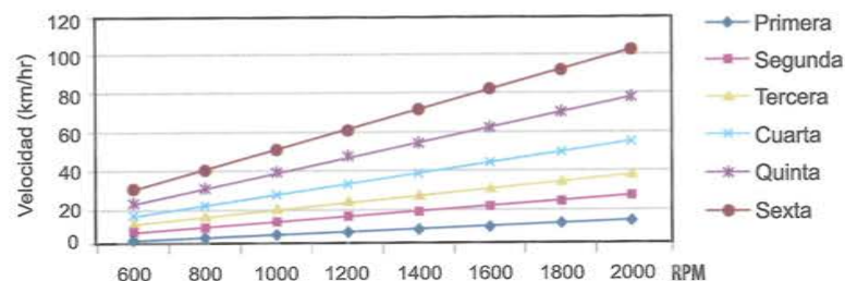
Diagrama de velocidades
