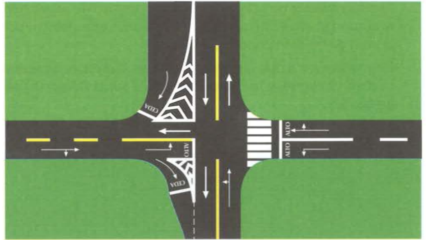
GRÁFICO 49: Alto y ceda.
