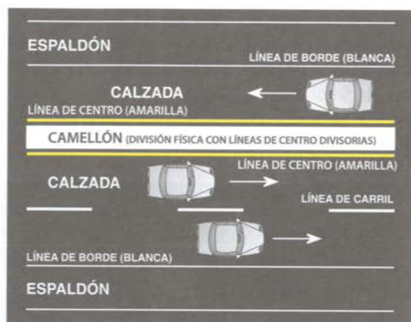
GRÁFICO 12: Línea de borde.
