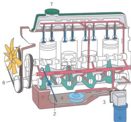
GRÁFICO 34: Sistema de lubricación.
