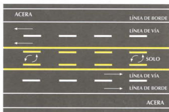
GRÁFICO 19: Carril exclusivo para giro a la izquierda.
