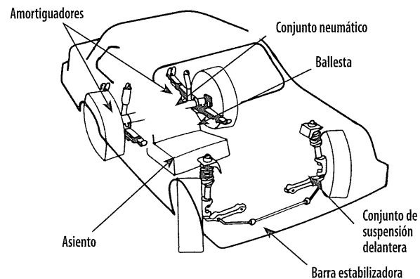
GRÁFICO 30: Sistema de suspensión y amortiguación.
